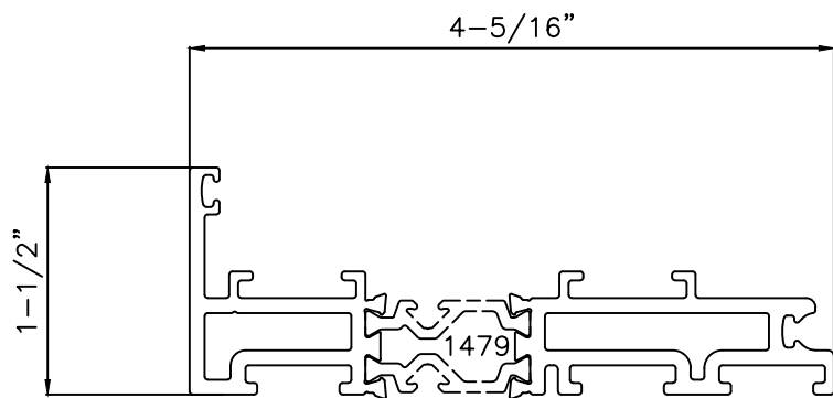
VENT 6063-T6
