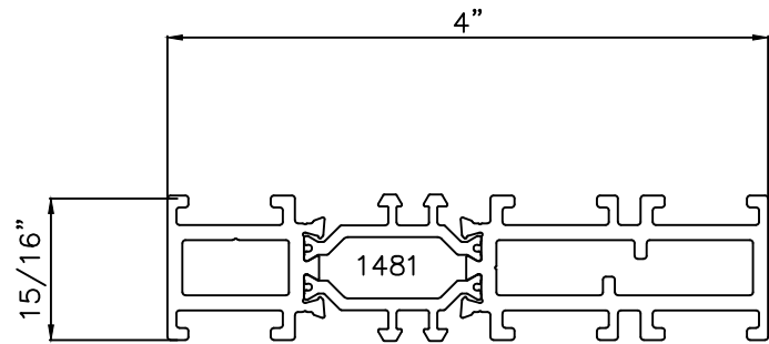
MASTER FRAME 6063-T6
