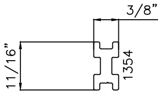
H-BAR 6063-T6
